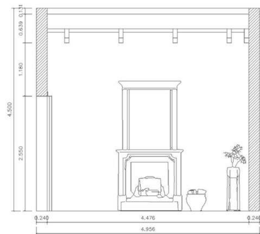
B Salle à manger B Façade 1:50
