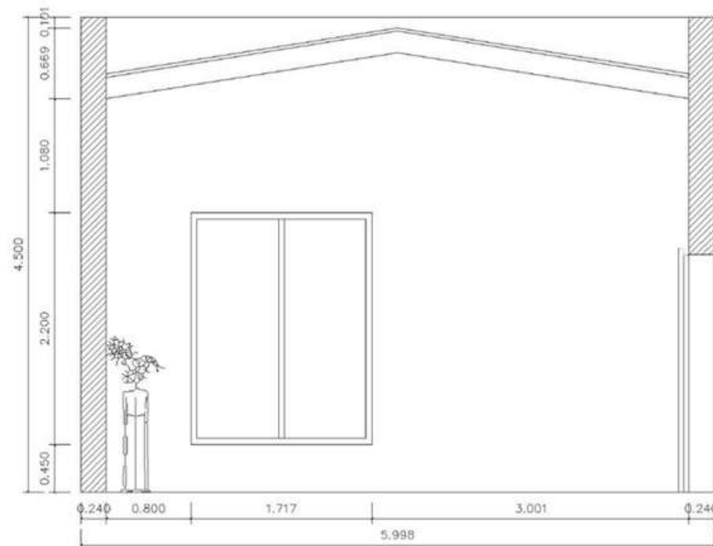
C Salle à manger C Façade 1:50
