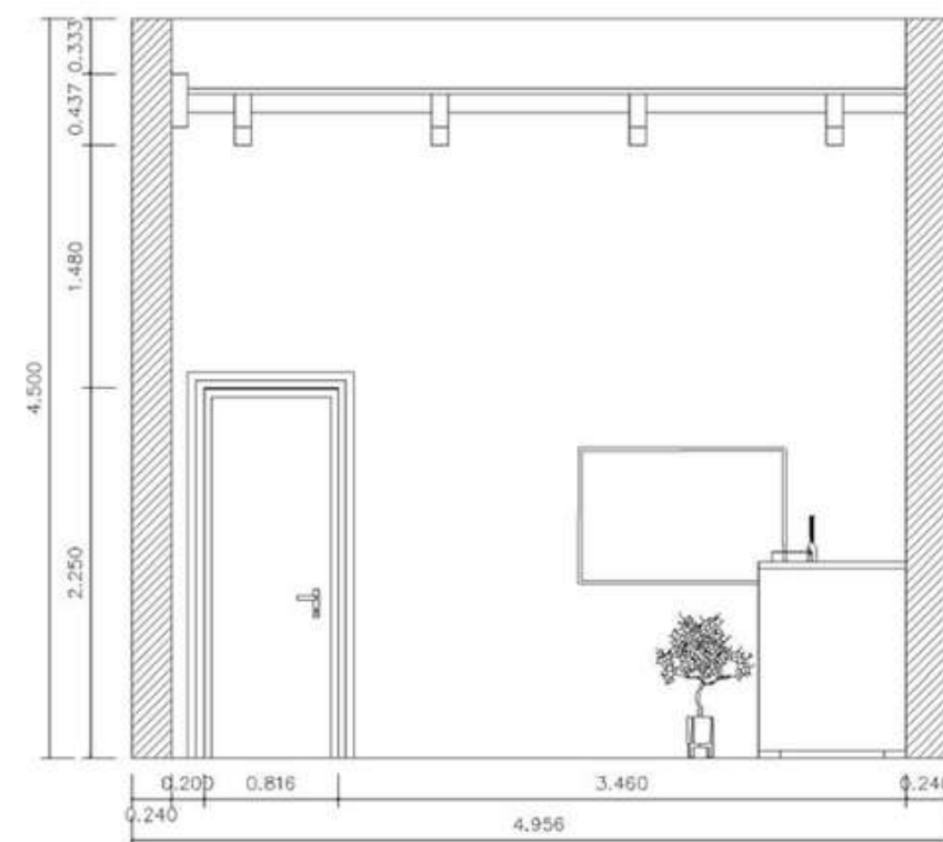
D Salle à manger D Façade 1:50
