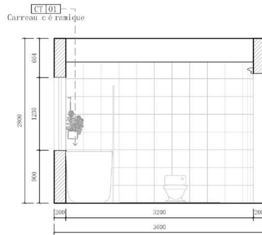
C Salle de bain C Façade 1:50
