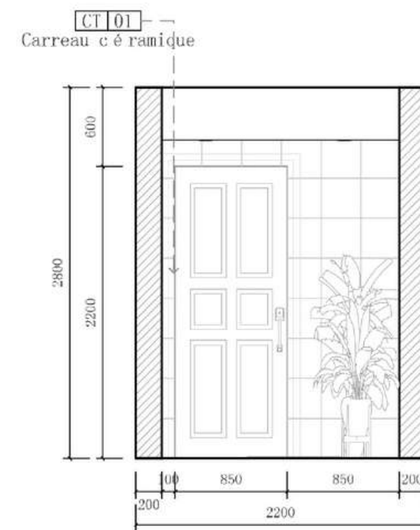
D Salle de bain D Façade 1:50
