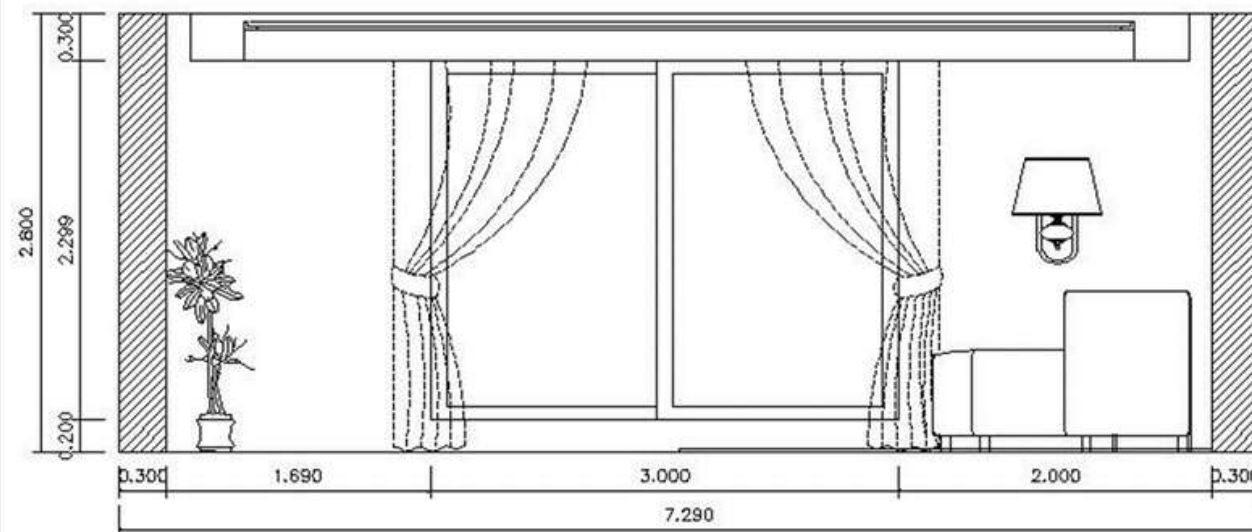
B B Salon Façade 1:50
