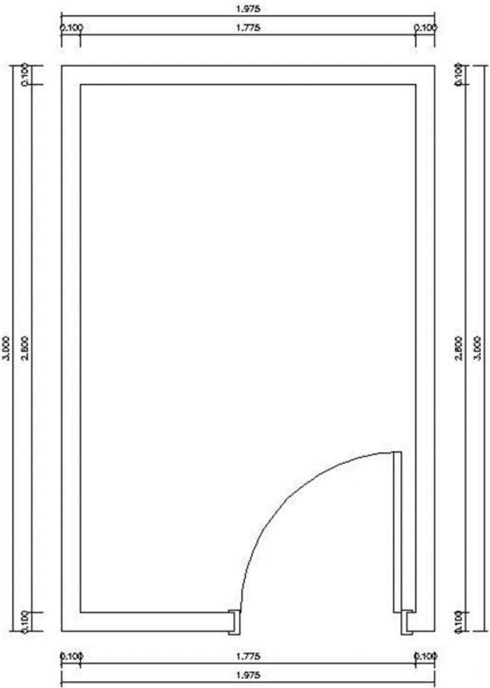
Plan 1:20
